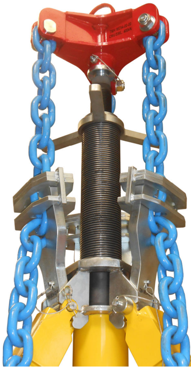
TMH ME94 test tool Outillage d'essai TMH ME94
